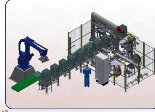
Otomatik Dizme Robot Konveyörü Auto Stacking Robot Conveyor
